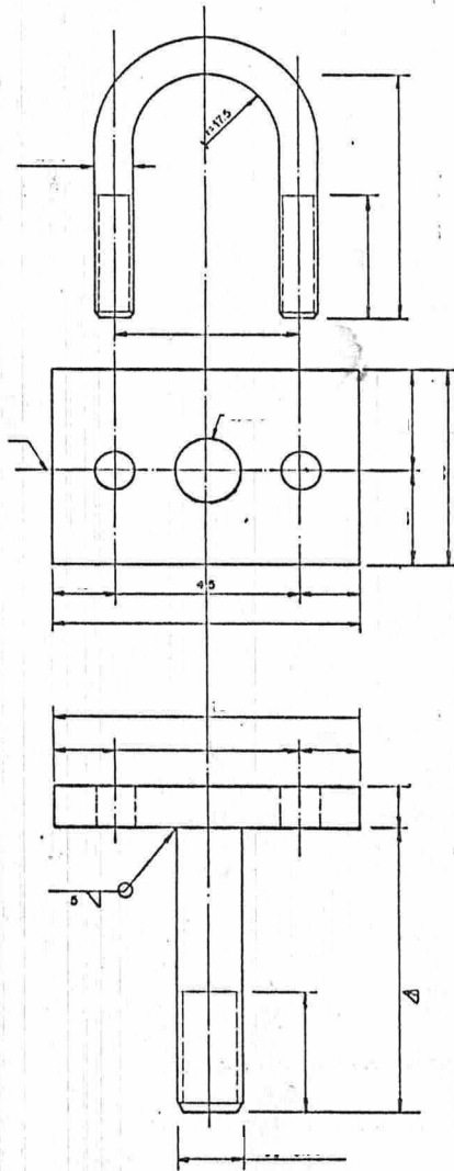
CONJUNTO SOPORTE "SC1"
